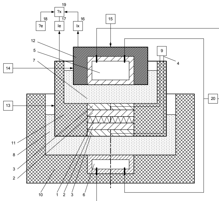
1 – джерело тепла; 2 – опорні взірці; 3 – температуровирівнюючі пластини; 4 – диференційна термопара; 5, 6 – приймачі тепла; 7 – досліджувана речовина; 8 – стандартна (порівняльна) речовина; 9 – нуль-індикатор; 10 – нерухома частина корпусу; 11, 12 – рухомі частини корпусу; 13, 14 – фіксуючі елементи; 15 – механізм переміщення; 16, 17 – вимірвальні перетворювачі переміщення; 18 – пристрій для задання коефіцієнта теплопровідності стандартної (порівняльної); 19 – мікропроцесорний пристрій; 20 – термостат
