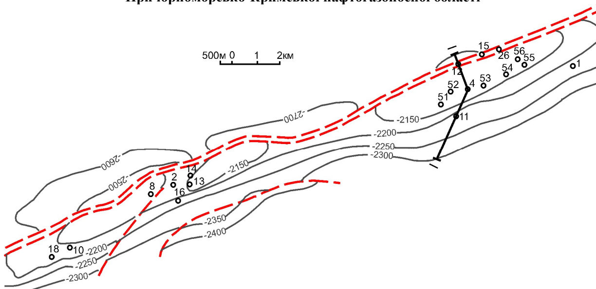
Рисунок 2 – Структурна схема покрівлі продуктивного горизонту П-ХІ (нижній палеоцен) (за О.Я.Дергачовою, 1987 р. з доповненнями С.М.Захарчука, 1994 р.)
