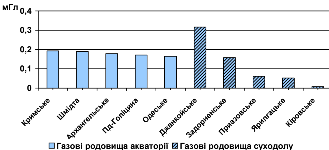
Рисунок 9 – Величина параметра гравітаційної контрастності для газових родовищ
