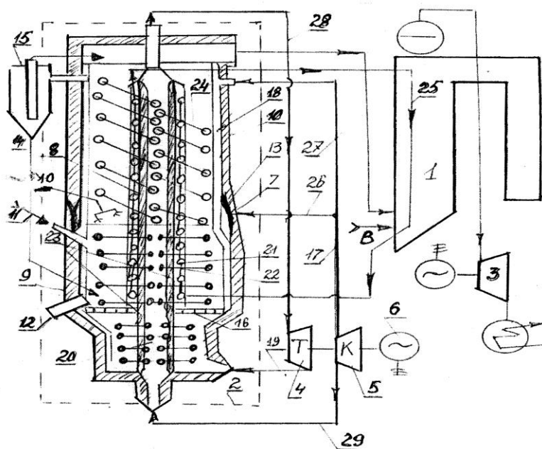
Рис.1. Парогазова енергетична установка з додатковою топкою киплячого шару
