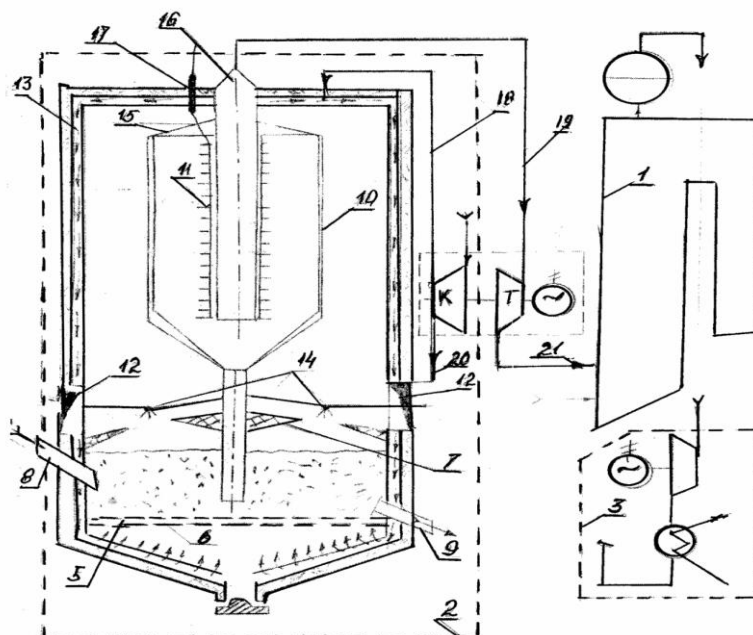
Рис. 2. Топка киплячого шару з вбудованим циклоном та високовольтним електрофільтром
