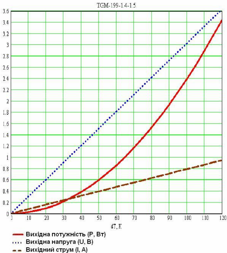
Рисунок 9 – Графіки залежності вихідних параметрів модуля TGM-199-1,4-1,5 від створеного перепаду температур на гарячій та холодній сторонах
