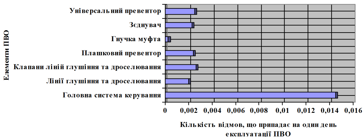
Рисунок 5 – Діаграма кількості відмов різних елементів ПВО, що припадає на один день експлуатації обладнання
